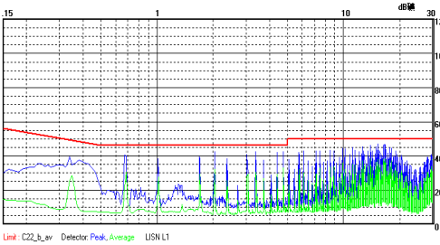
VRB2405YMD-6WR2 传导骚扰 Class B 测试效果图 (正线)
