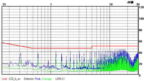
VRA2415YMD-6WR2 传导骚扰 Class B 测试效果图 (正线)
