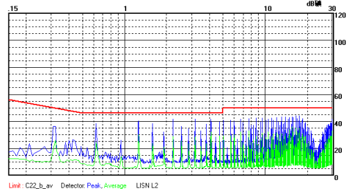
VRA2415YMD-6WR2 传导骚扰 Class B 测试效果图 (负线)
