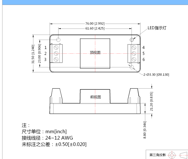
外观尺寸
