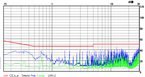
VRB2405YMD-6WR2 传导骚扰 Class B 测试效果图 (负线)
