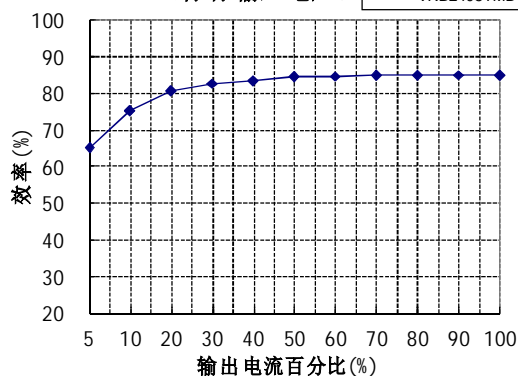
效率VS输出负载曲线图
