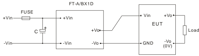
标称电压小于 48V 时, C \geq 330\mu\text{F}/50\text{V} 标称电压等于 48V 时, C \geq 330\mu\text{F}/100\text{V} FT-A/BX1D 为我司脉冲群抑制器, 具体型号请参照选型手册。 图 3
